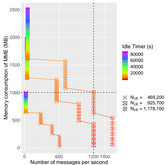
図 7 Idle タイマに対する、メッセージ処理頻度とメモリ使用量の関係 (シナリオ 2, N_{UE} = 469,200, 925,700, 1,178,100 )
