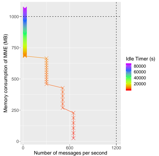
図 6 Idle タイマに対する、メッセージ処理頻度とメモリ使用量の関係 (シナリオ 2)
